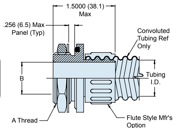
Type B Conduit Adapter Style 5
